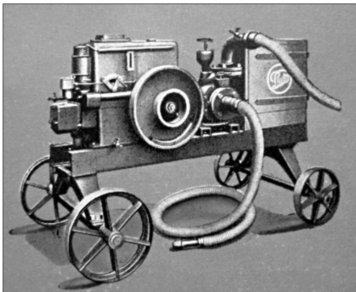
Požární stříkačka. Firemní leták
