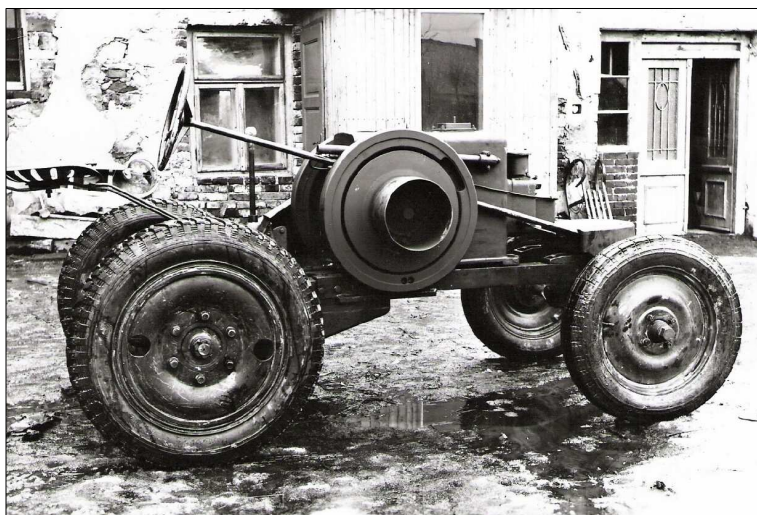
Čtyřkolový traktor Pluto. Archiv J. Štefánka
