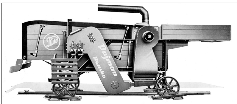
Mlātička značky Minima. Firemní leták
