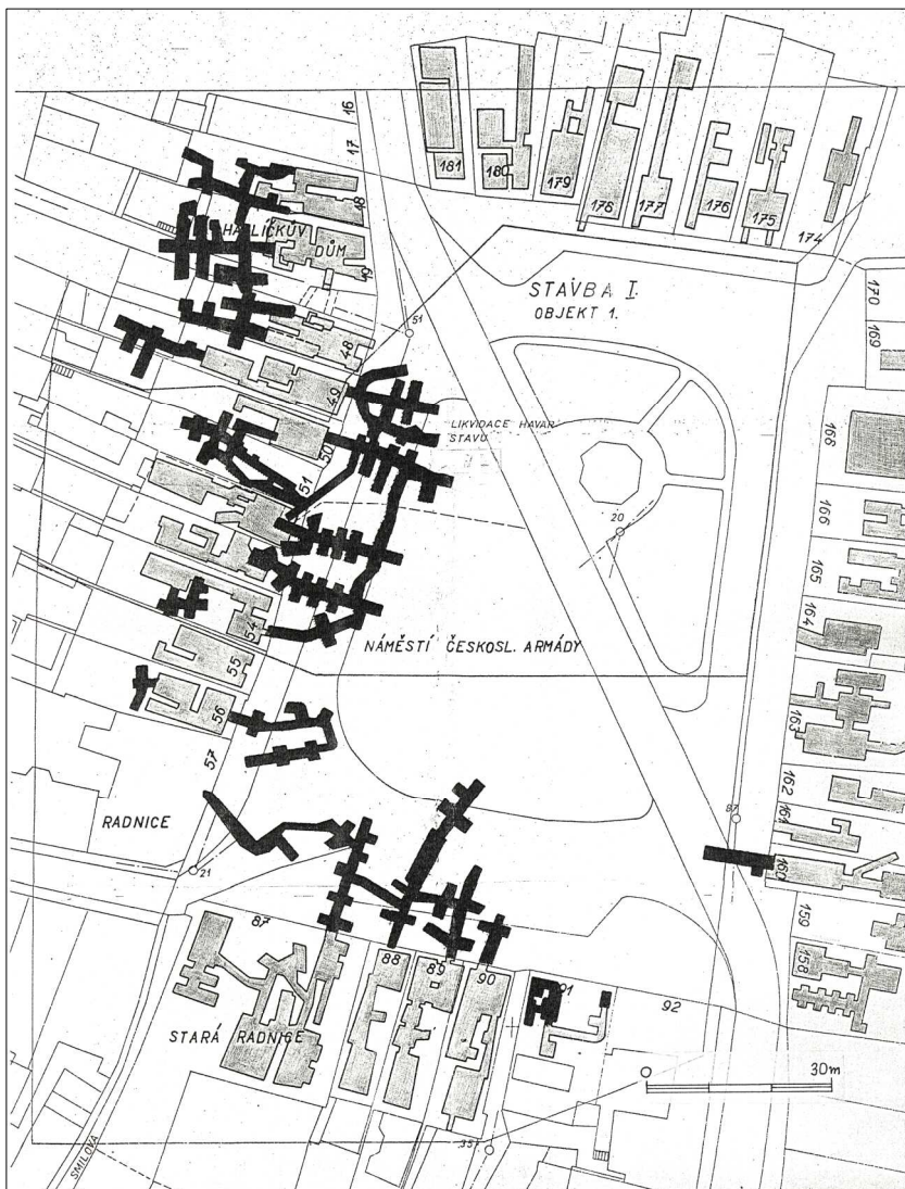
Obr. č. 1 - Situace podzemních chodeb (vyznačeny černě) a sklepů (šedě) měšťanských domů na Havlíčkově náměstí zjištěná inženýrsko-geologickým průzkumem v období kolem roku 1968. Upraveno podle výkresu č. 8.
