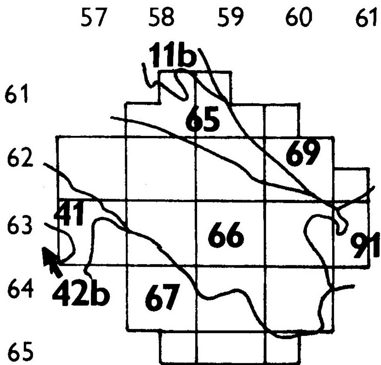
obr. 2 Fytogeografické členění území (11b – Poděbradské Polabí, 41 – Střední Povltaví, 42b – Táborsko-vlašimská pahorkatina, 65 – Kutnohorská pahorkatina, 66 – Hornosázavská pahorkatina, 67 – Českomoravská vrchovina, 69 – Železné hory, 91 – Žďárské vrchy).
